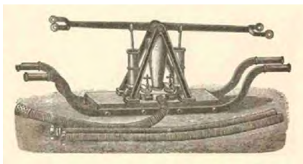
Пожарная труба (ручной пожарный насос) – это переносной насос двойного действия (всасывающего и нагнетательного), предназначенный для целей пожаротушения
